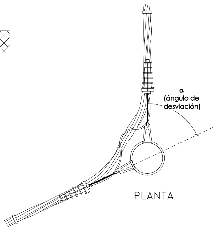
DETALLE 1
