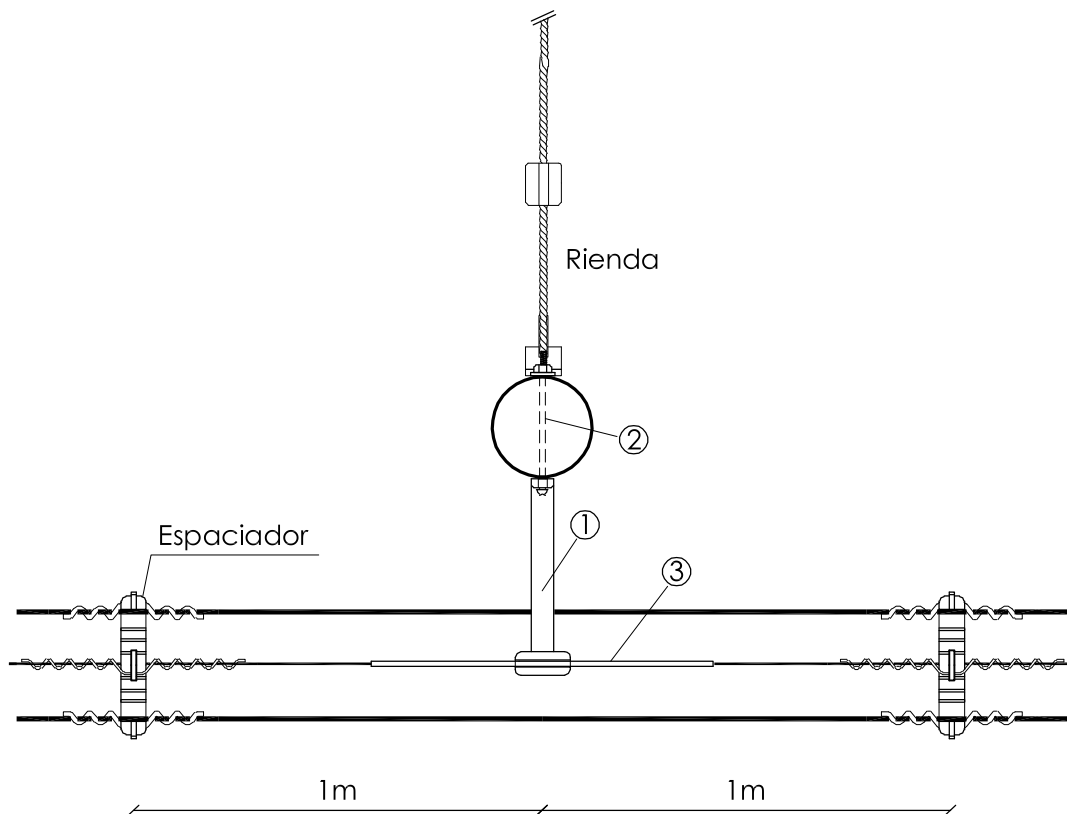
VISTA SUPERIOR
