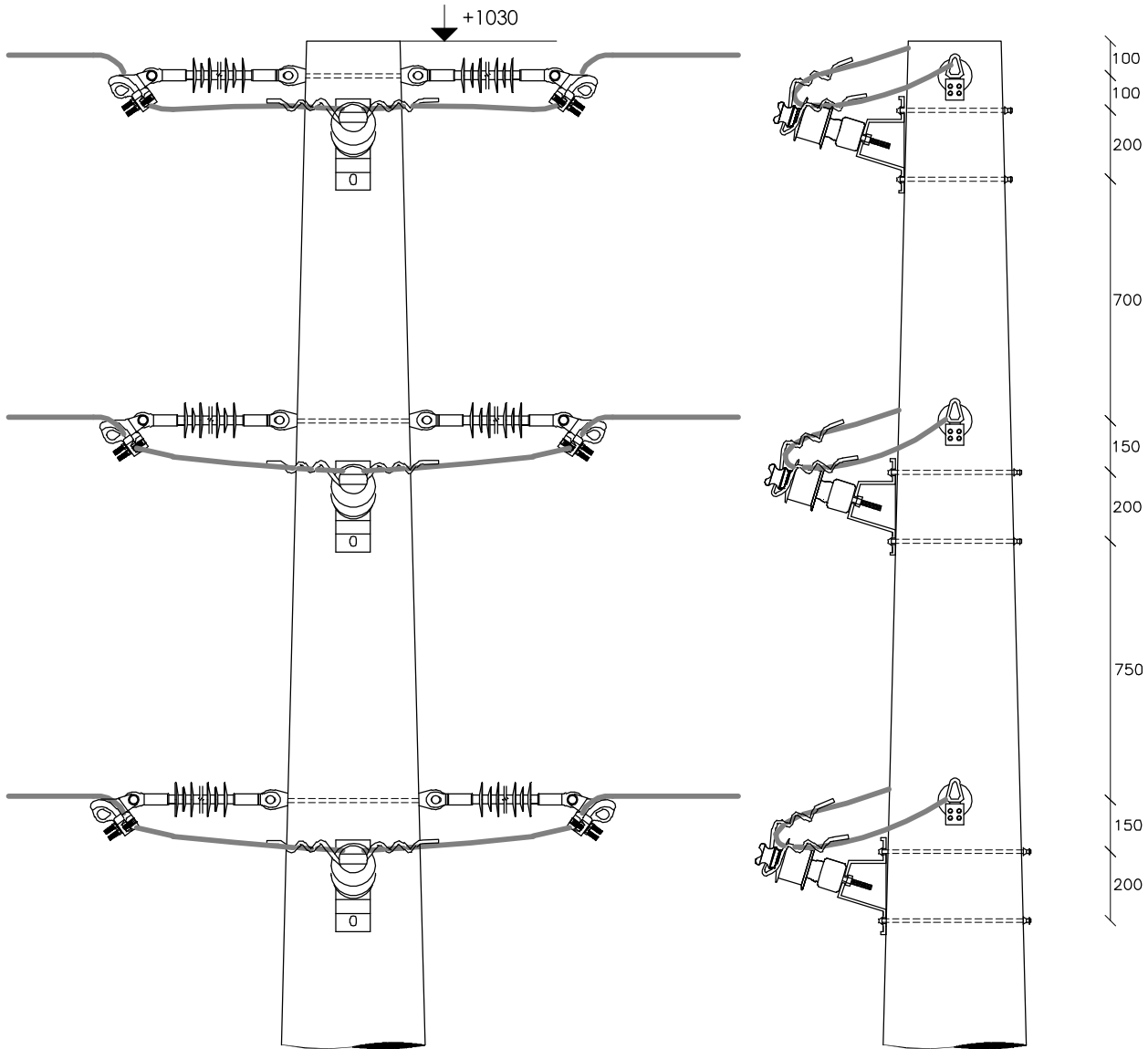
ALZADO FRONTAL
